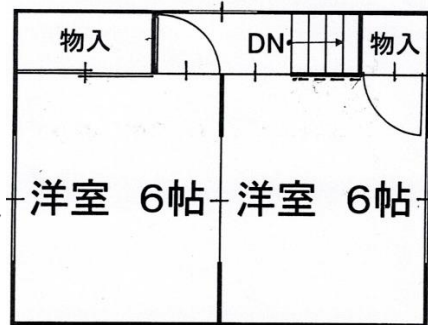
2階平面図
